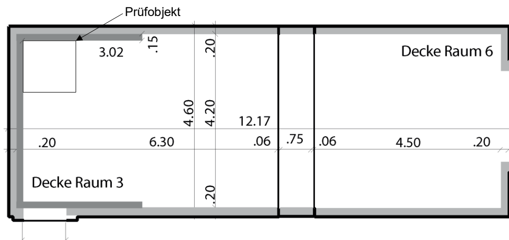
Abbildung 2: Grundriss des Prüfstands mit Positionierung des Prüfobjekts auf der Decke von Raum 3
