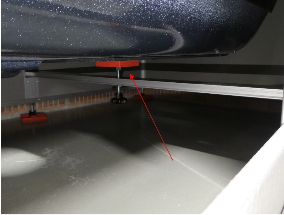
Abbildung 5: Detailansicht innen von Prüfaufbau 1 mit Abstützung der Wanne mittig über dasselbe entkoppelnde Element
