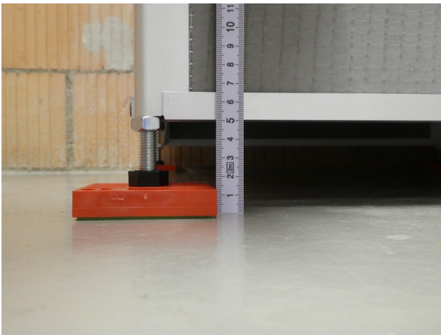
Abbildung 4: Prüfaufbau 1 mit Metermass
