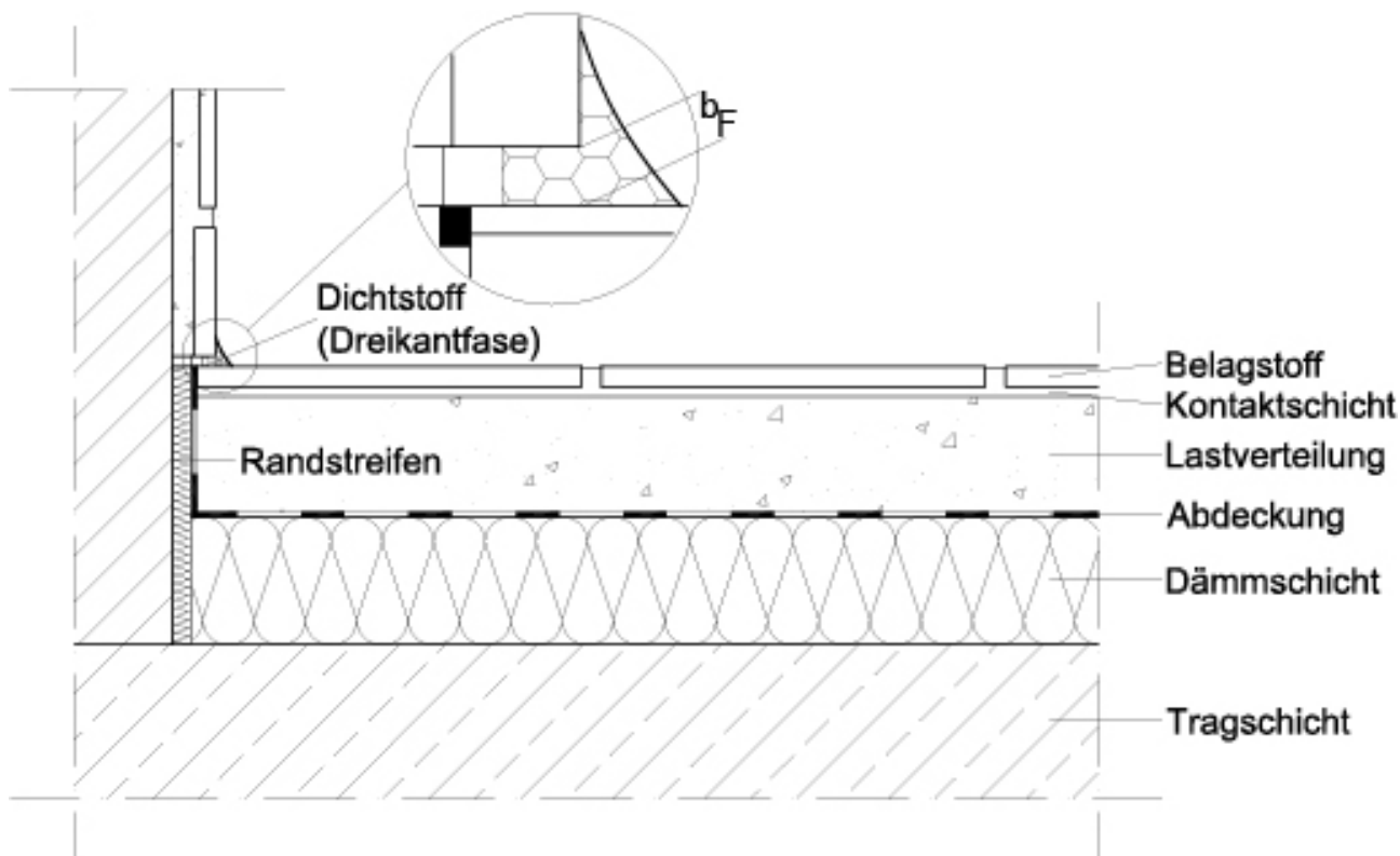
Abbildung 2: Dreiecksfuge (Dreikantfase)
