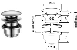
Ventil für clic-clack – Waschbecken mit verchromtem Verzierungerring / Ecoulement pour clic-clack – Lavabos avec anneau décoratif chromé
