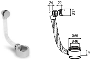
Überlauf für Waschbecken / Trop-plein pour lavabos
