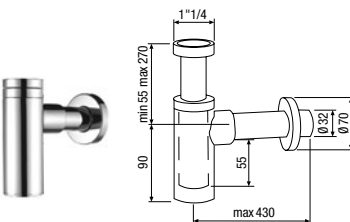
Verchromter Siphon für Waschbecken, runder Querschnitt / Siphon chromé pour lavabos, section transversale ronde
