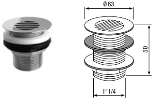
Ventil für Waschbecken mit Gitter, ohne Chromverschluss / Bonde pour lavabo avec grille, sans fermeture chromée
