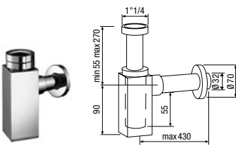
Verchromter Siphon für Waschbecken, eckiger Querschnitt / Siphon chromé pour lavabos, section transversale carrée
